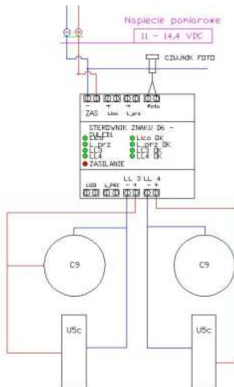
Rys. 4. Układ podłączenia znaków do sterownika
