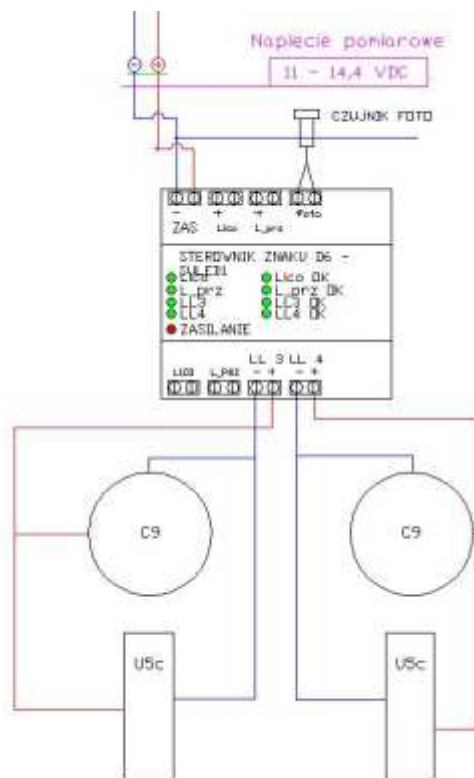
Rys. 8. Układ podłączenia znaków do sterownika
