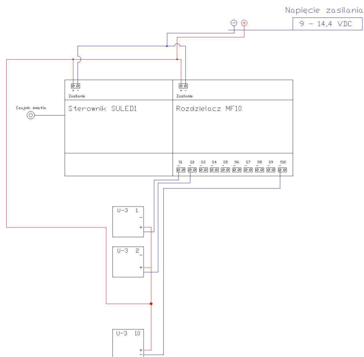
Rys. 6. Układ podłączenia znaków do sterownika
