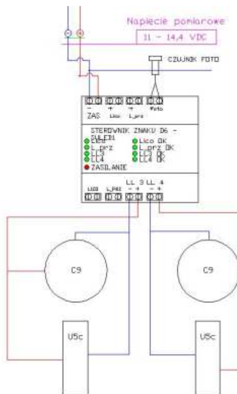
Rys. 10. Układ podłączenia znaków do sterownika
