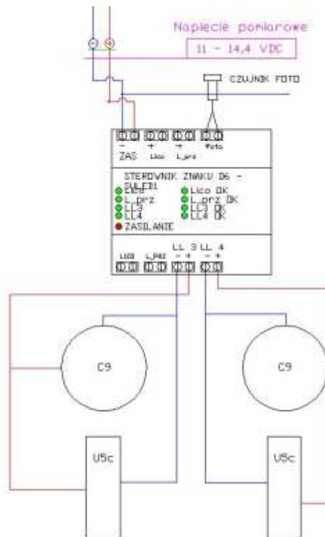
Rys. 8. Układ podłączenia znaków do sterownika
